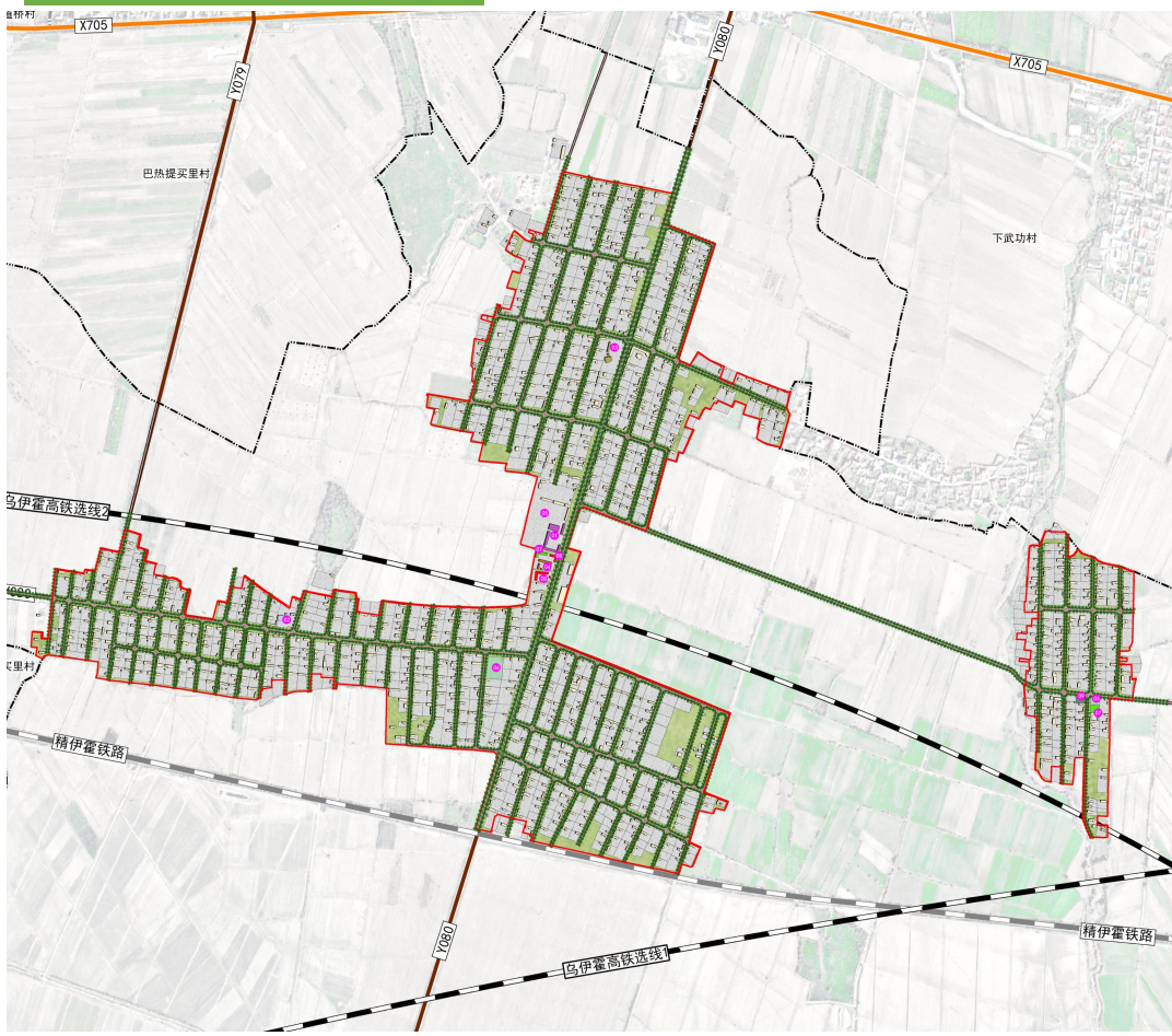
规划总平面图
